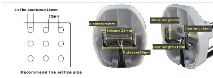
SF1001- Orifice Plate
